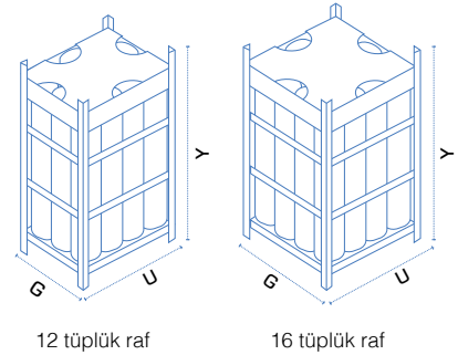
12 tüplük raf
